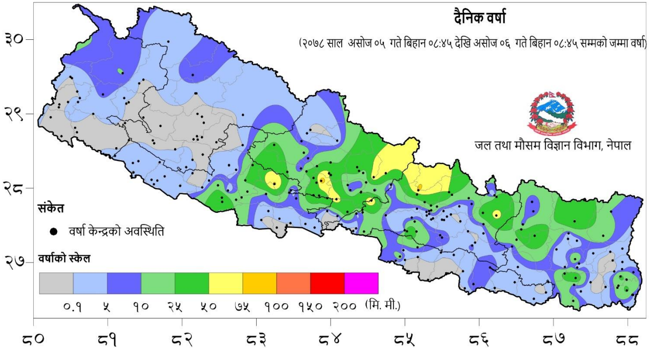
नक्सा १: असोज ०५ गते बिहान ०८:४५ बजे देखि असोज ०६ गते बिहान ०८:४५ बजे सम्मको २४ घण्टाको वर्षा (मि. मी.)
