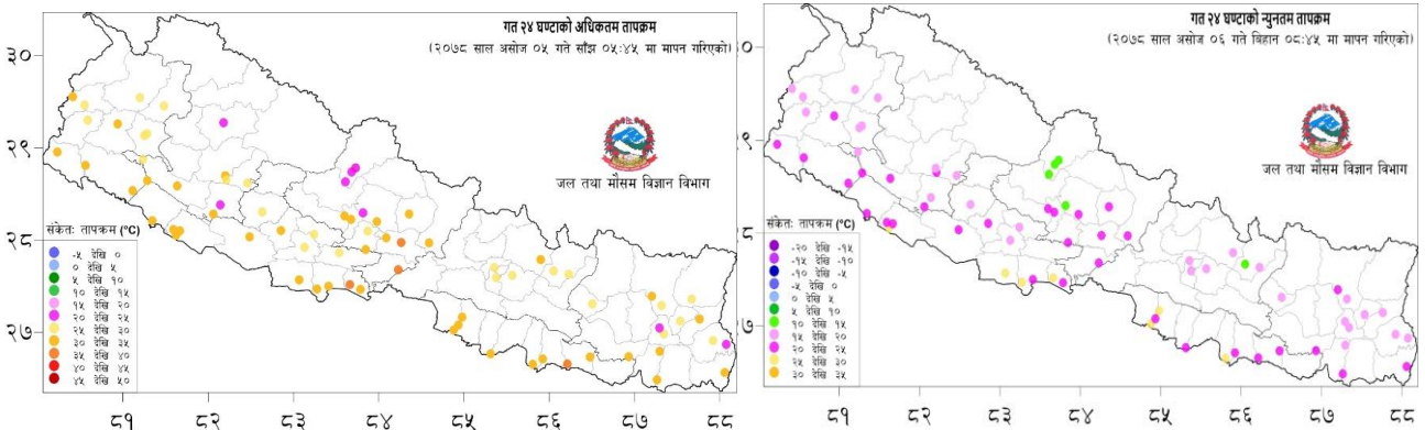
नक्सा ३: असोज ०४ गते साँझ ०५:४५ बजे देखि गते असोज ०५ साँझ ०५:४५ बजे सम्मको २४ घण्टाको अधिकतम तापक्रम (डिग्री सेल्सियस)
