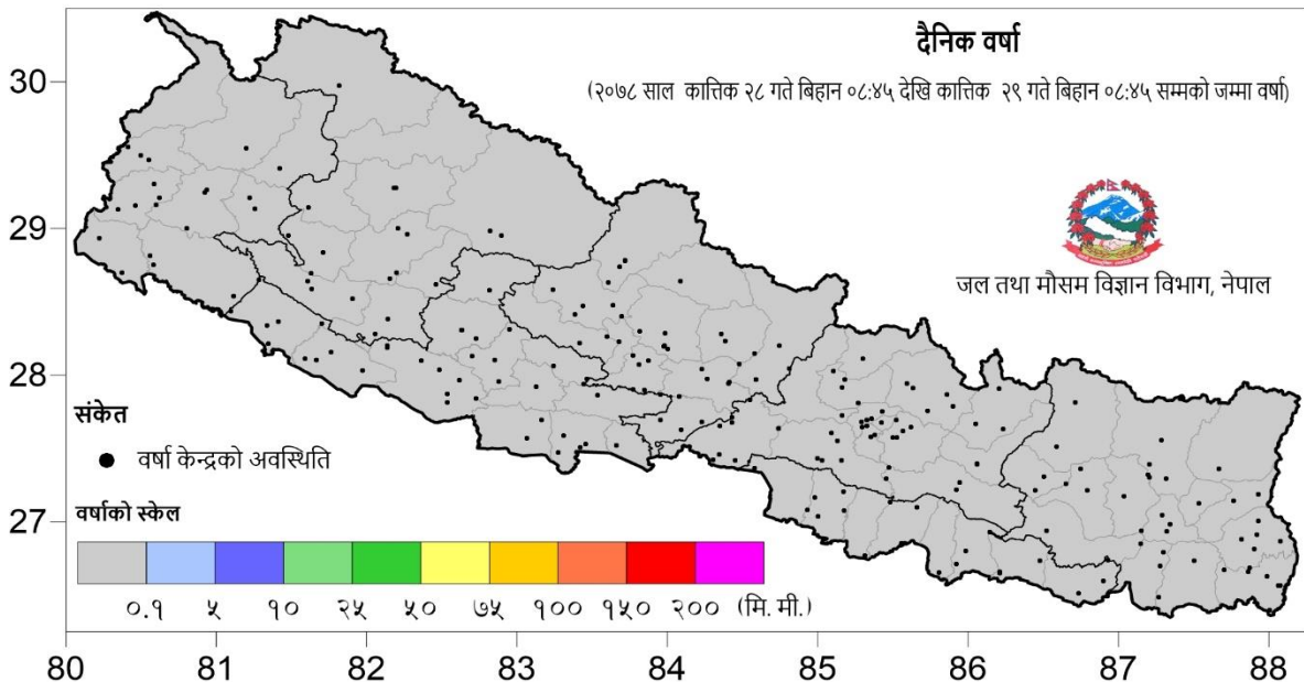
नक्सा १: कार्तिक २८ गते बिहान ०८:४५ बजे देखि कार्तिक २९ गते बिहान ०८:४५ बजे सम्मको २४ घण्टाको वर्षा (मि. मी.)
