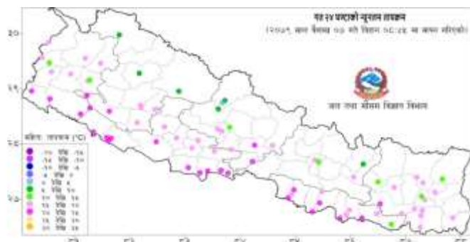
नक्सा २: वैशाख ०६ गते बिहान ०८:४५ बजे देखि वैशाख ०७ गते बिहान ०८:४५ बजे सम्मको २४ घण्टाको न्यूनतम तापक्रम (डिग्री सेल्सियस)
