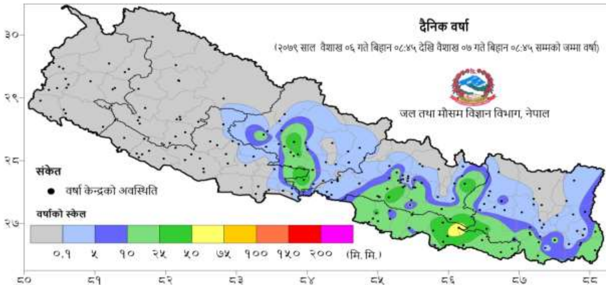
नक्सा १: वैशाख ०६ गते बिहान ०८:४५ बजे देखि वैशाख ०७ गते बिहान ०८:४५ बजे सम्मको २४ घण्टाको वर्षा (मि. मि.)
