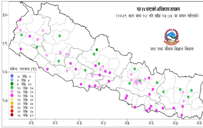
नक्सा २: माघ ०३ गते साँझ ०५:४५ बजे देखि माघ ०४ गते साँझ ०५:४५ बजे सम्मको २४ घण्टाको अधिकतम तापक्रम (डिग्री सेल्सियस)
