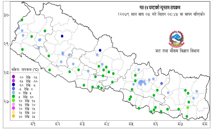
नक्सा ३: माघ ०४ गते बिहान ०८:४५ बजे देखि माघ ०५ गते बिहान ०८:४५ बजे सम्मको २४ घण्टाको न्यूनतम तापक्रम (डिग्री सेल्सियस)
