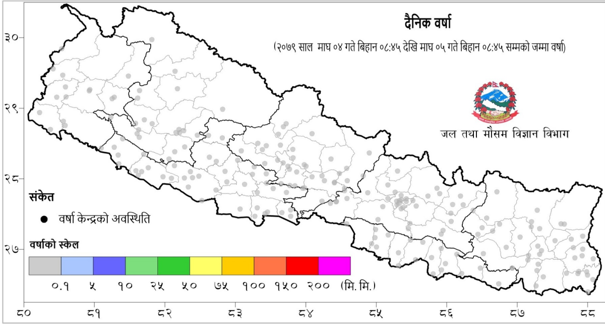
नक्सा १: माघ ०४ गते बिहान ०८:४५ बजे देखि माघ ०५ गते बिहान ०८:४५ बजे सम्मको २४ घण्टाको वर्षा (मि. मि.)
