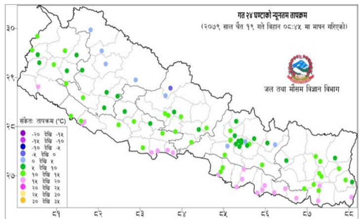
नक्सा ३: चैत १८ गते बिहान ०८:४५ बजे देखि चैत १९ गते बिहान ०८:४५ बजे सम्मको २४ घण्टाको न्यूनतम तापक्रम (डिग्री सेल्सियस)
