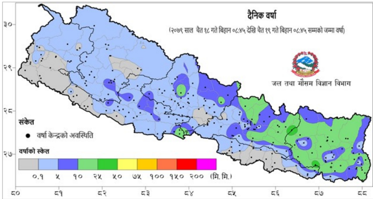
नक्सा १: चैत १८ गते बिहान ०८:४५ बजे देखि चैत १९ गते बिहान ०८:४५ बजे सम्मको २४ घण्टाको वर्षा (मि. मि.)
