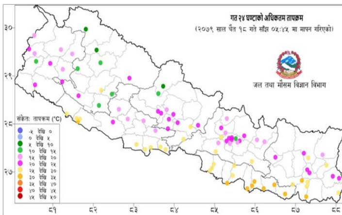
नक्सा २: चैत १७ गते साँझ ०५:४५ बजे देखि चैत १८ गते साँझ ०५:४५ बजे सम्मको २४ घण्टाको अधिकतम तापक्रम (डिग्री सेल्सियस)
