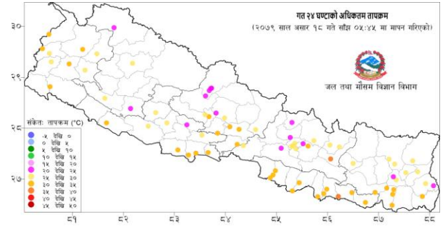
नक्सा ३: असार १७ गते साँझ ०५:४५ बजे देखि असार १८ गते साँझ ०५:४५ बजे सम्मको २४ घण्टाको अधिकतम तापक्रम (डिग्री सेल्सियस)
