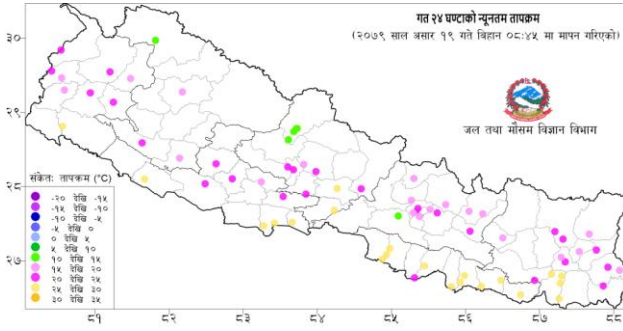
नक्सा २: असार १८ गते बिहान ०८:४५ बजे देखि असार १९ गते बिहान ०८:४५ बजे सम्मको २४ घण्टाको न्यूनतम तापक्रम (डिग्री सेल्सियस)
