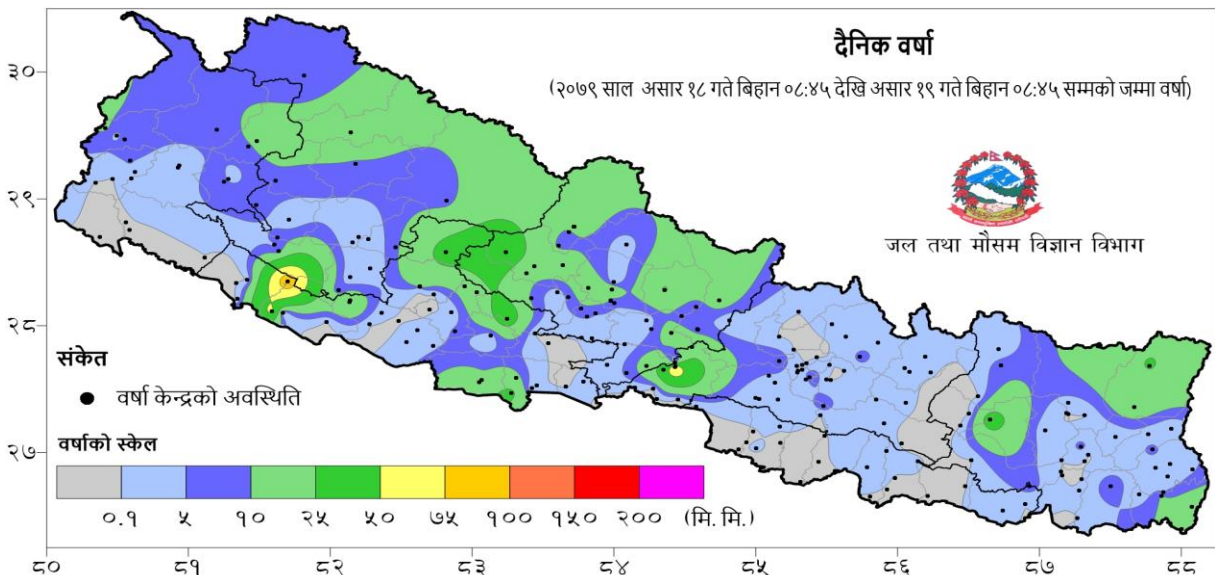
नक्सा १: असार १८ गते बिहान ०८:४५ बजे देखि असार १९ गते बिहान ०८:४५ बजे सम्मको २४ घण्टाको वर्षा (मि. मि.)
