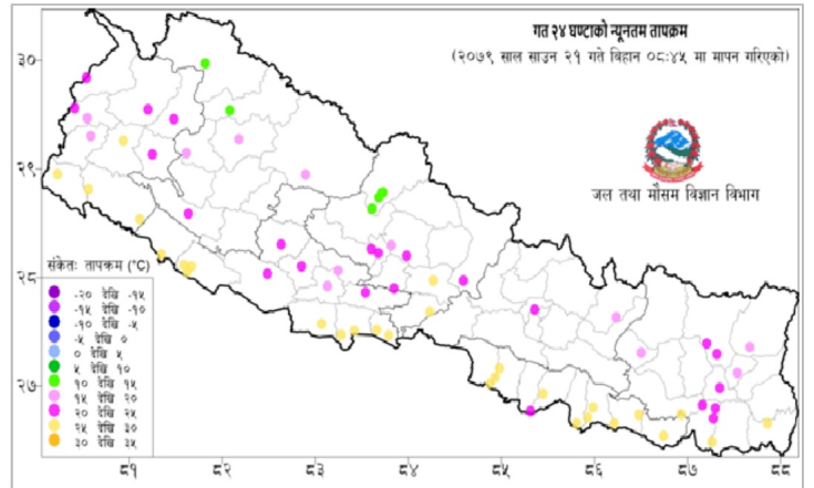
नक्सा ३: साउन २० गते बिहान ०८:४५ बजे देखि साउन २१ गते बिहान ०८:४५ बजे सम्मको २४ घण्टाको न्यूनतम तापक्रम (डिग्री सेल्सियस)
