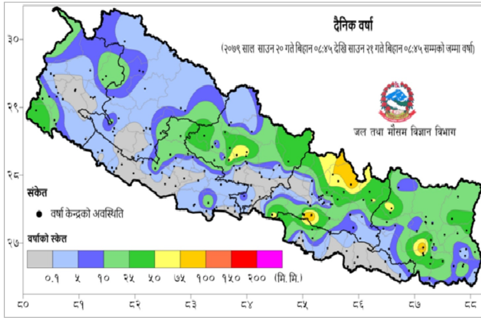
नक्सा १: साउन २० गते बिहान ०८:४५ बजे देखि साउन २१ गते बिहान ०८:४५ बजे सम्मको २४ घण्टाको वर्षा (मि. मि.)
