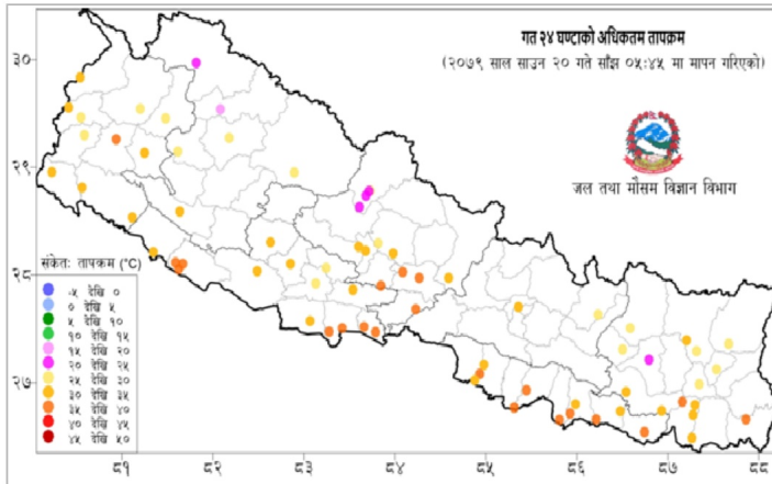
नक्सा २: साउन १९ गते साँझ ०५:४५ बजे देखि साउन २० गते साँझ ०५:४५ बजे सम्मको २४ घण्टाको अधिकतम तापक्रम (डिग्री सेल्सियस)
