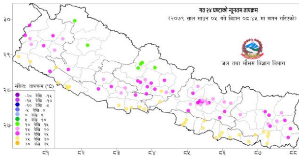
नक्सा २: साउन ०४ गते बिहान ०८:४५ बजे देखि साउन ०५ गते बिहान ०८:४५ बजे सम्मको २४ घण्टाको न्यूनतम तापक्रम (डिग्री सेल्सियस)
