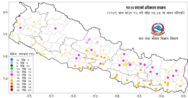
नक्सा ३: साउन ०३ गते साँझ ०५:४५ बजे देखि साउन ०४ गते साँझ ०५:४५ बजे सम्मको २४ घण्टाको अधिकतम तापक्रम (डिग्री सेल्सियस)
