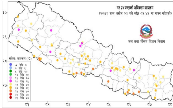
नक्सा २: असोज ०२ गते साँझ ०५:४५ बजे देखि असोज ०३ गते साँझ ०५:४५ बजे सम्मको २४ घण्टाको अधिकतम तापक्रम (डिग्री सेल्सियस)
