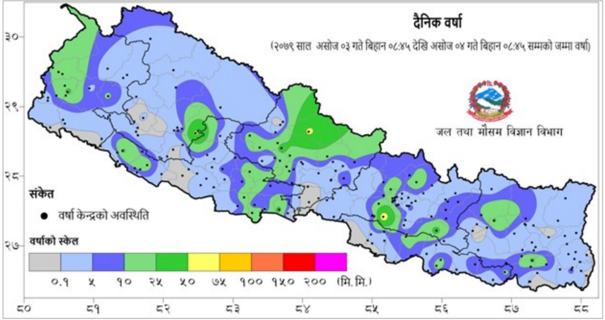
नक्सा १: असोज ०३ गते बिहान ०८:४५ बजे देखि असोज ०४ गते बिहान ०८:४५ बजे सम्मको २४ घण्टाको वर्षा (मि. मि.)
