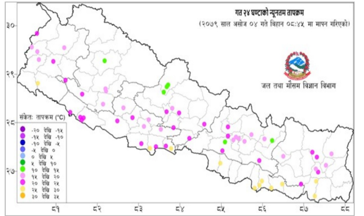
नक्सा ३: असोज ०३ गते बिहान ०८:४५ बजे देखि असोज ०४ गते बिहान ०८:४५ बजे सम्मको २४ घण्टाको न्यूनतम तापक्रम (डिग्री सेल्सियस)
