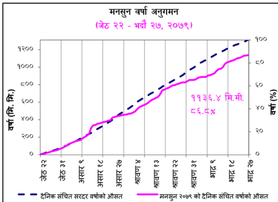
चित्र नं. २: २० वटा मौसम केन्द्रहरू (नक्सा १ को गोलाकार संकेत) मा मापन गरिएको मनसुन अवधिको दैनिक सञ्चित सरदर वर्षाको औसत (नीलो रंगको खण्डित रेखा) र सन् २०२२ जुन ५ देखि सेप्टेम्बर १२ (वि.सं. २०७९ जेठ २२ देखि भदौ २७) सम्मको १०० दिनको संचित वर्षाको औसत (गुलाबी रेखा)
