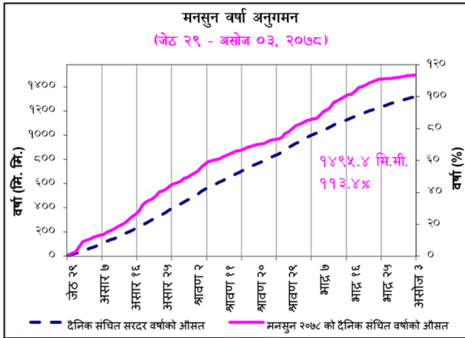
चित्र नं. १: २० वटा मौसम केन्द्रहरू (नक्सा १ को गोलाकार संकेत) मा मापन गरिएको मनसुन अवधिको दैनिक सञ्चित सरदर वर्षाको औसत (नीलो रंगको खण्डित रेखा) र सन् २०२१ जुन १२ देखि सेप्टेम्बर १९ (वि.सं. २०७८ जेठ २९ देखि असोज ०३) सम्मको १०० दिनको संचित वर्षाको औसत (गुलाबी रेखा)
