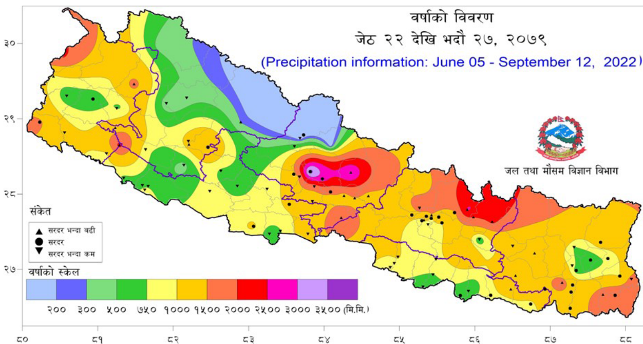
चित्र नं. ४: पृष्ठभूमिको रंगले मनसुन शुरु भए देखि १०० दिन सम्म (जेठ २२ देखि भदौ २७, २०७९) को जम्मा वर्षा (मि.मि.) देखाउँदछ। माथि तिर चुच्चो भएको त्रिभुजले सर्दर भन्दा बढी वर्षा भएको, गोलाकारले सर्दर वर्षा भएको र तलतिर चुच्चो भएको त्रिभुजले सर्दर भन्दा कम वर्षा भएको केन्द्रलाई जनाउँदछ।
